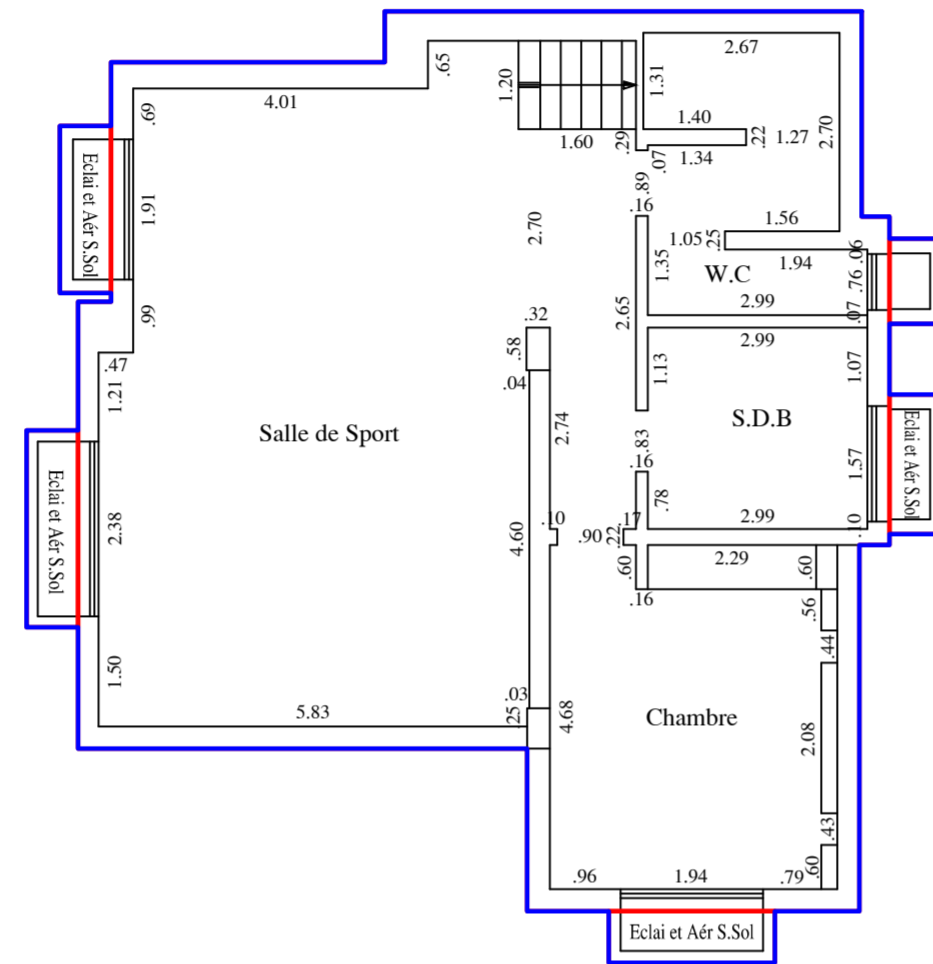
SOUS SOL
