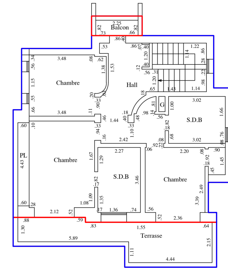
1er ETAGE
